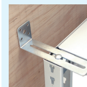
【支柱上部止め】 A・B金具使用
